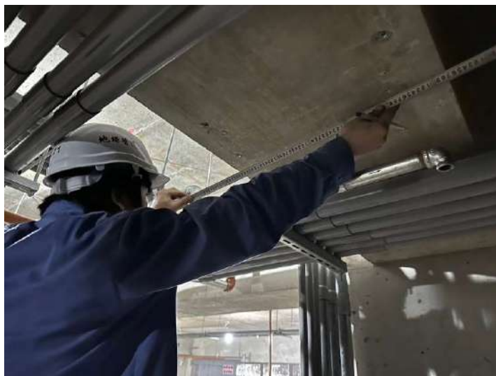
B1F消防管配管
