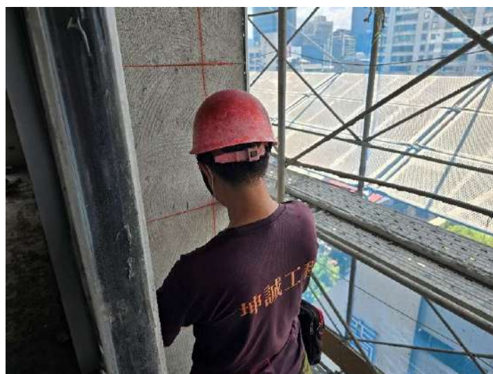
10F外牆磁磚放樣
