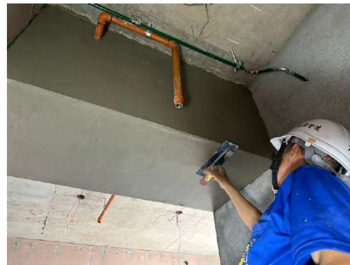
11F室內打底施作
