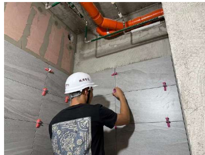
4F浴廁磁磚施作
