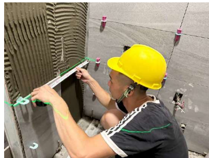
6F浴廁磁磚施作
