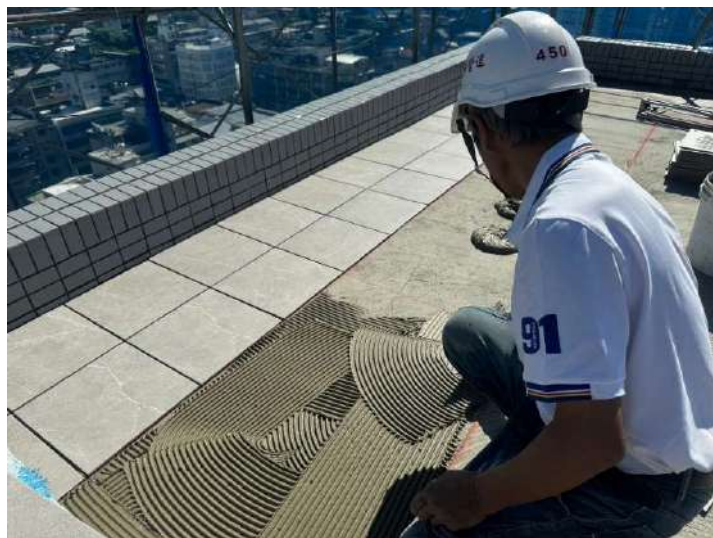
屋頂版地磚施作
