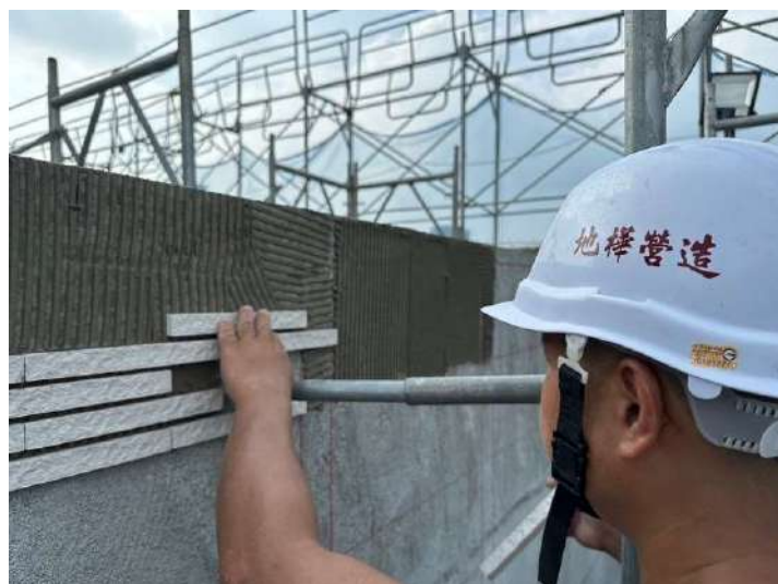
R1西側外牆長條磚施作
