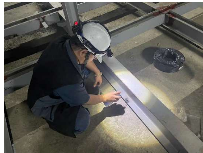
停車設備骨架焊接處除鏽噴漆
