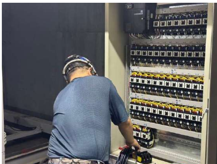
停車設備控制盤電源配線
