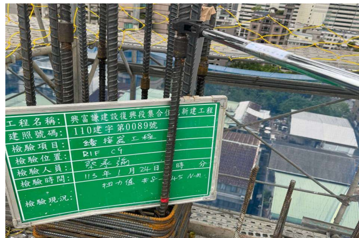
柱筋查驗
