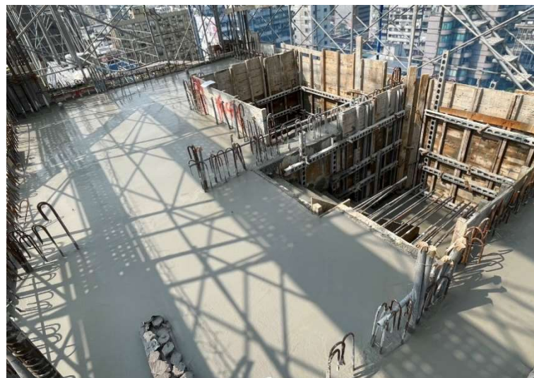
R2F 版灌漿完成
