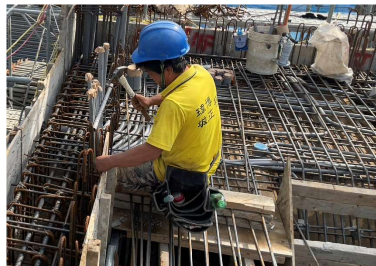
R1F 樓梯組模
