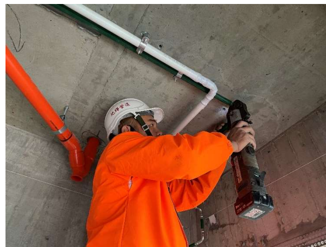
給水管壓接施作
