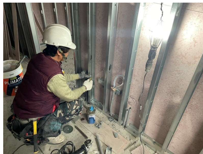
輕隔間配管
