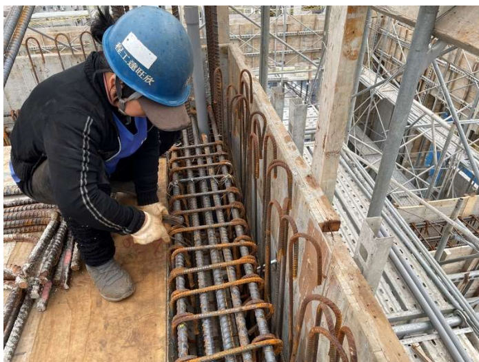
R3F 樑筋綁紮
