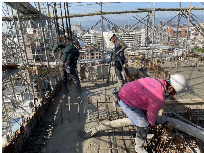
R3F 版灌漿
