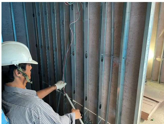
隔間配管作
