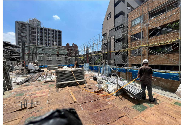
灌漿後以麻布袋養護混凝土
