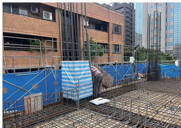
柱頭鋪設帆布保護，避免灌漿汙染
