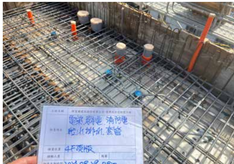
機電配管查驗
