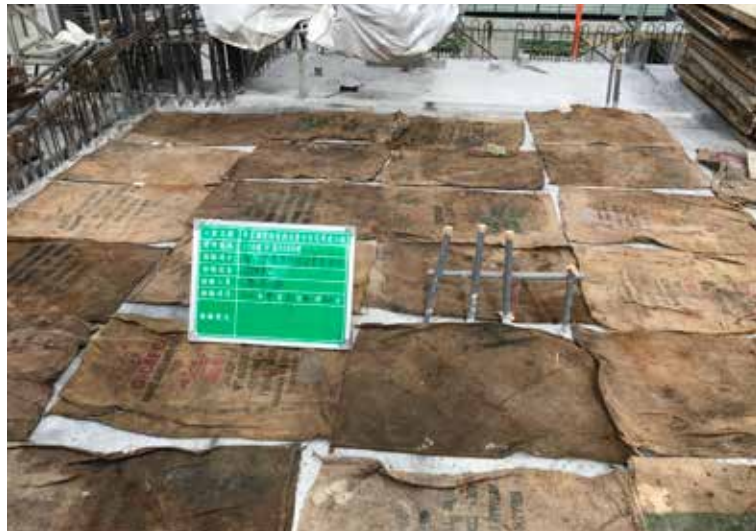
灌漿後鋪設麻布袋灑水養護
