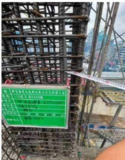
柱筋彎鉤查驗
