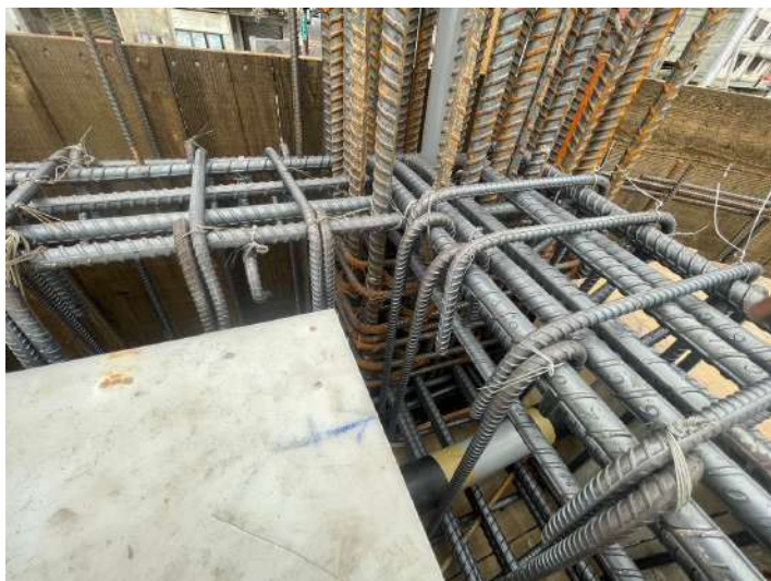
二樓版樑鋼筋綁紮
