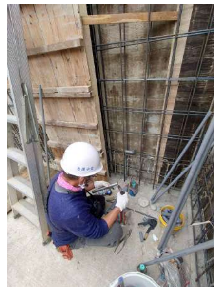
水電牆面配管
