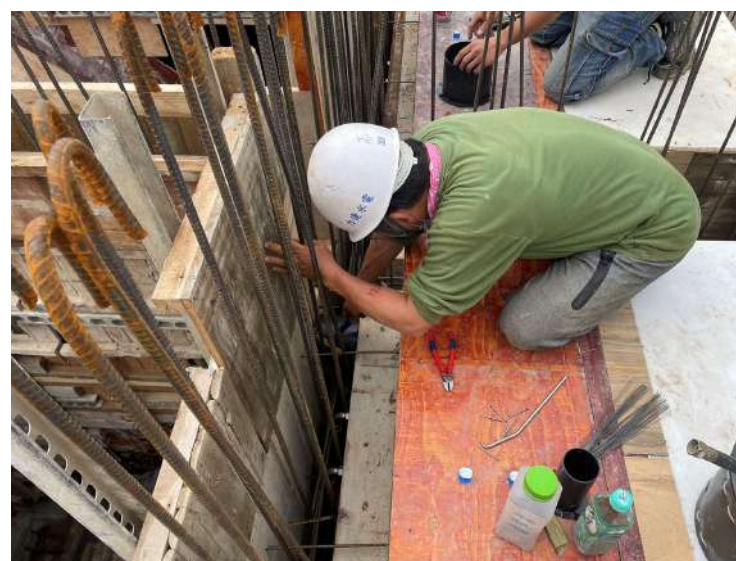
三樓版水電施工
