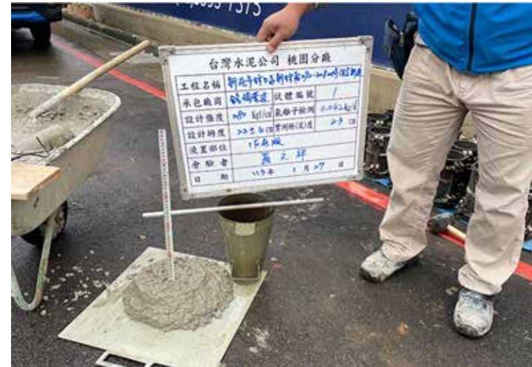
混凝土坍度檢測
