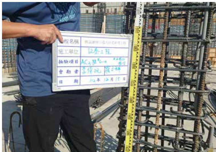
柱筋查驗
