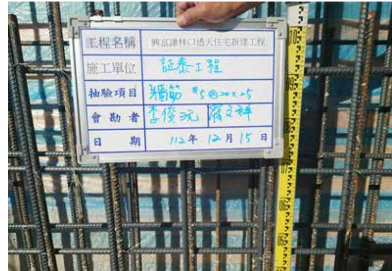
鋼筋查驗(2)
