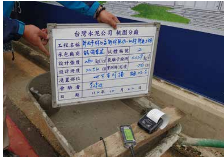
混凝土氯離子檢測
