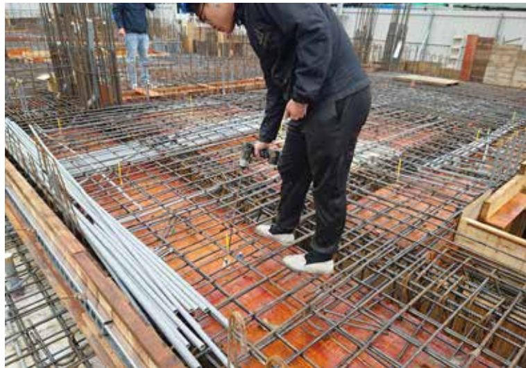
標高器施作
